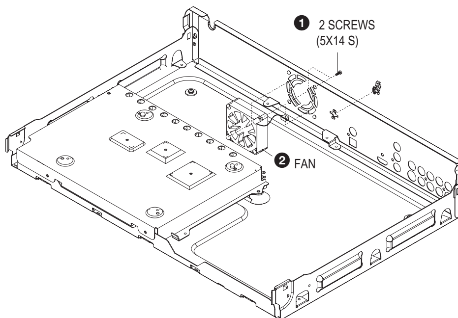
Fig. 3-6 FAN Removal
